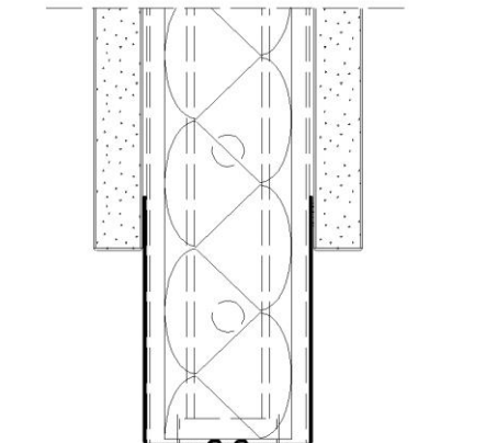
Vollbeplankung M 1:2
